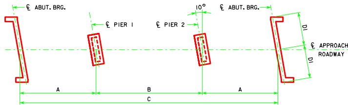
10° SKEW (R.A.)
