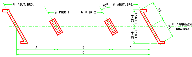
30° SKEW (R.A.)
