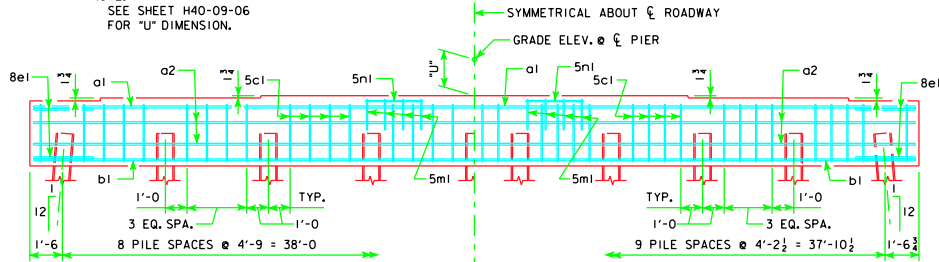
9 PILE BENT
