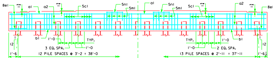
13 PILE BENT
