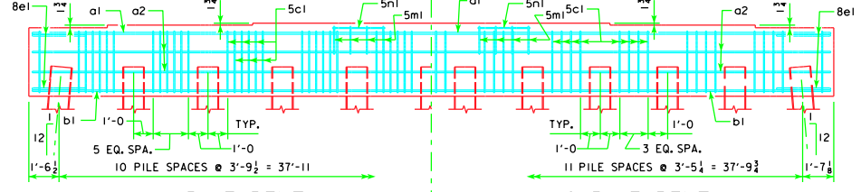
11 PILE BENT
