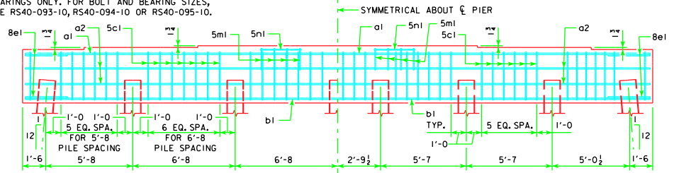
7 PILE BENT
