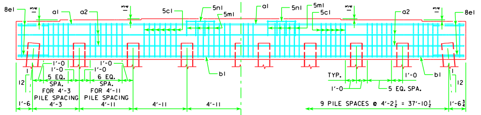
9 PILE BENT
