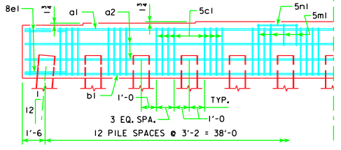
13 PILE BENT
