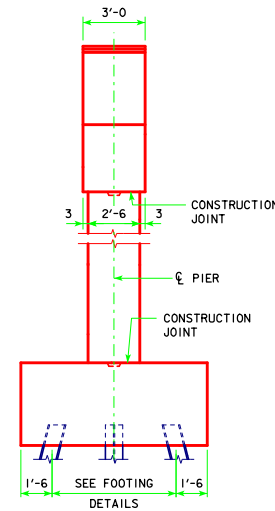
END ELEVATION
