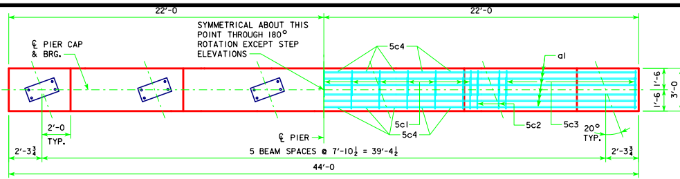
CAP PLAN
