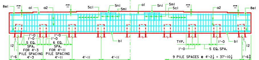
9 PILE BENT
