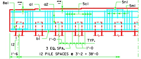
13 PILE BENT
