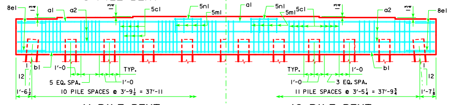
11 PILE BENT
