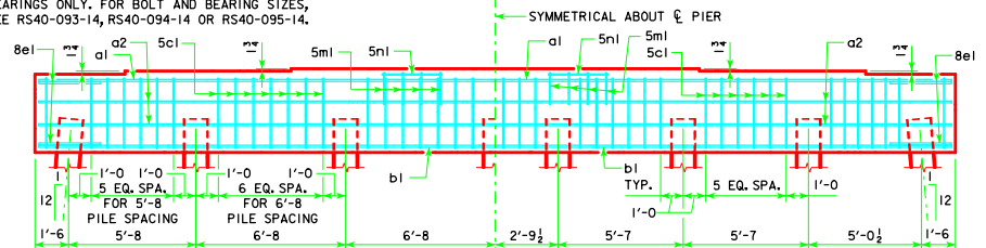
7 PILE BENT
