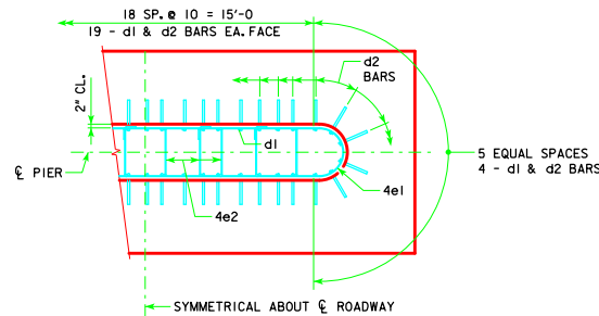
d2 BAR LAYOUT
