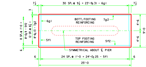
3'-6 x 9'-0 x 25'-0
