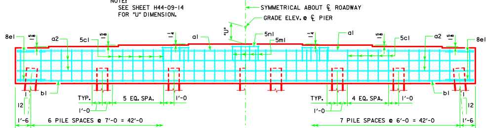
7 PILE BENT
