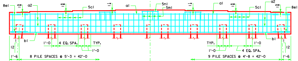
9 PILE BENT
