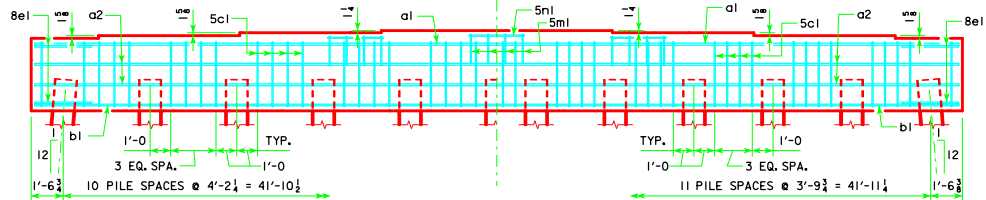
11 PILE BENT
