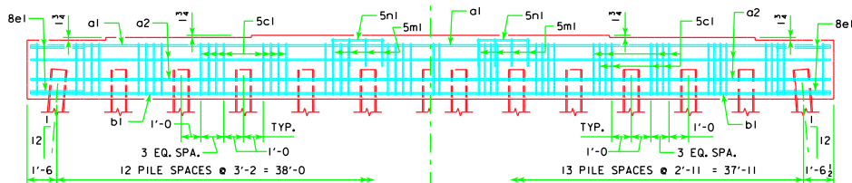
13 PILE BENT
