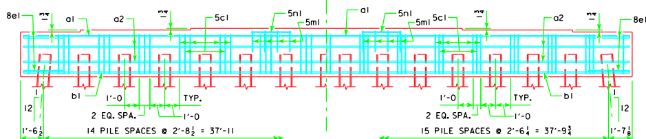
15 PILE BENT
