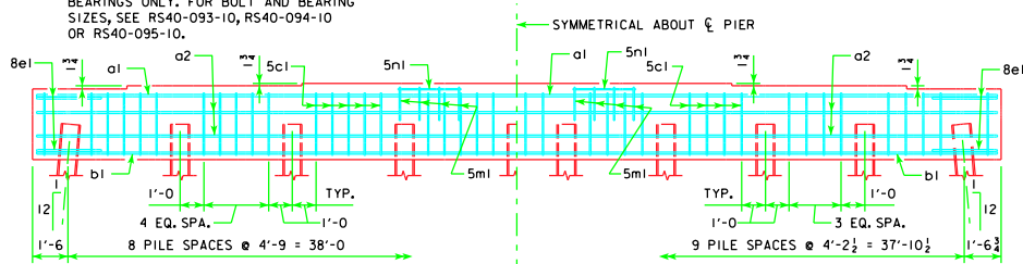
9 PILE BENT
