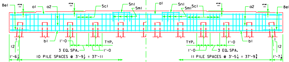
11 PILE BENT
