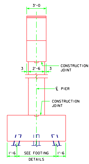
END ELEVATION
