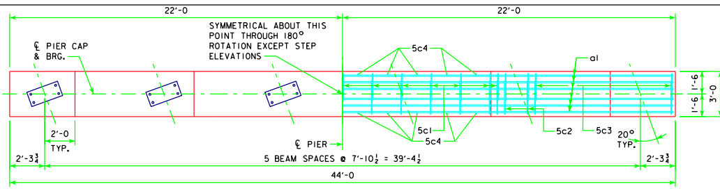
CAP PLAN
