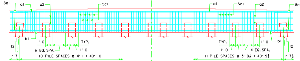
11 PILE BENT
