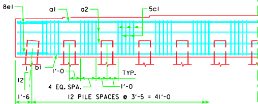
13 PILE BENT
