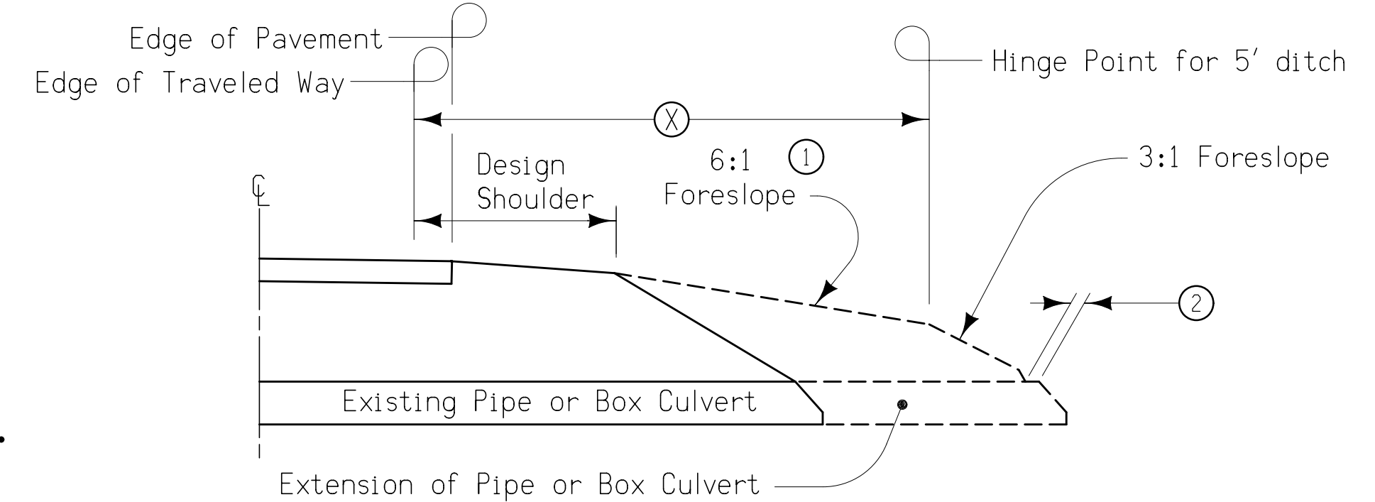
SECTION A-A
