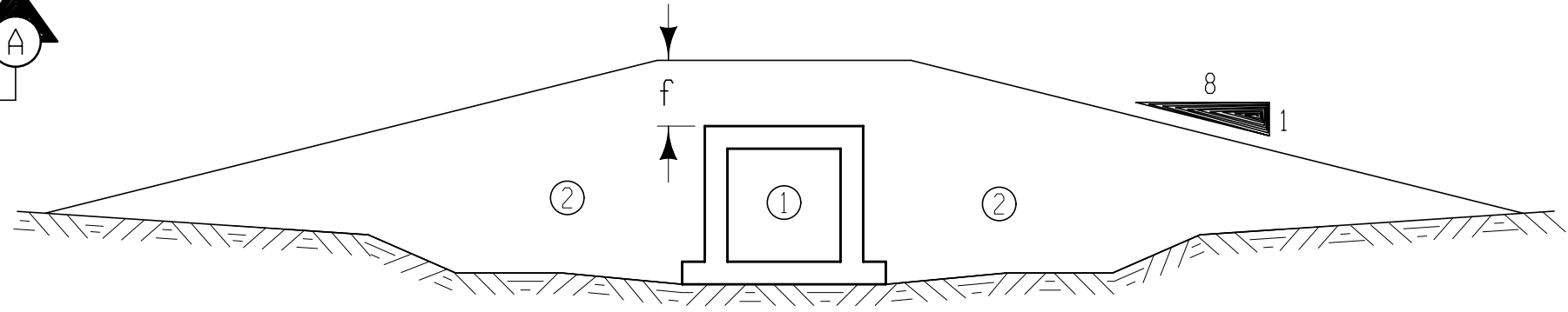
SECTION A-A
